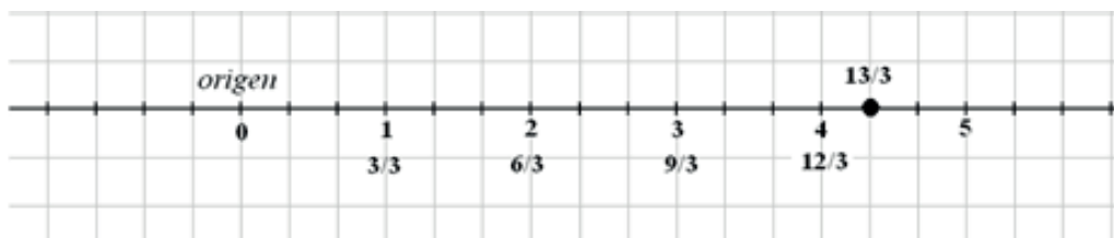
Figura 2.11. Localización de trece tercios.
