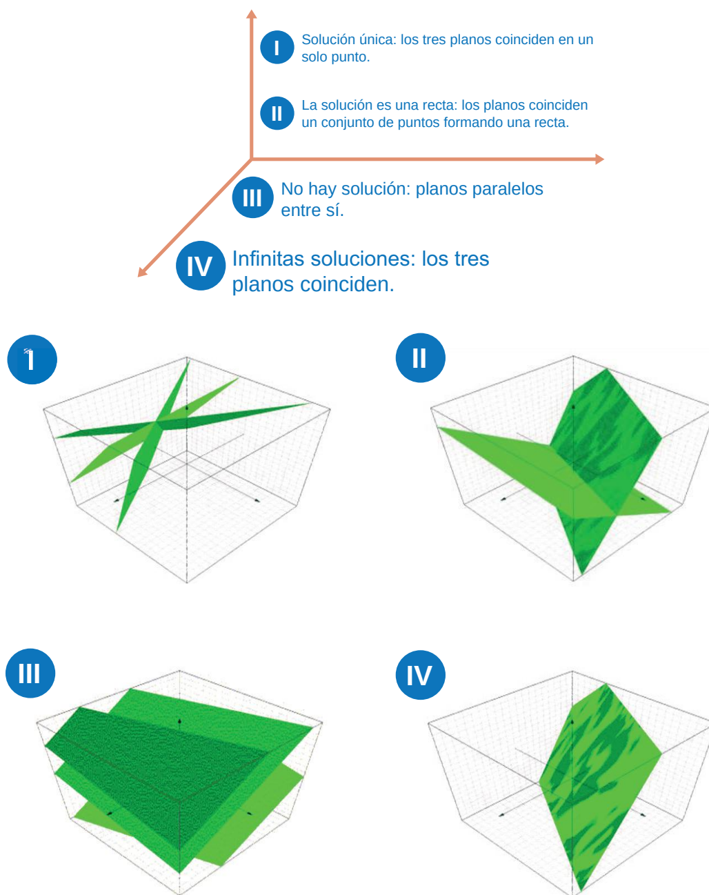
Figura 8.7. Soluciones de un sistema lineal 3 \times 3 .
